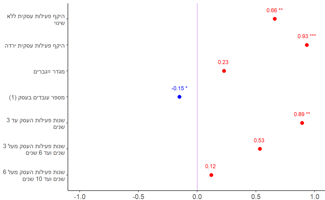
(1) משתנה מספר עובדים בעסק בקבוצות של 10, 1-10, 11-20 מאפייני המודל הסטטיסטי
